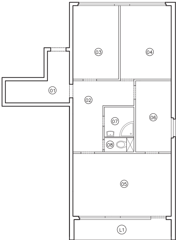
bytová jednotka 686/01
