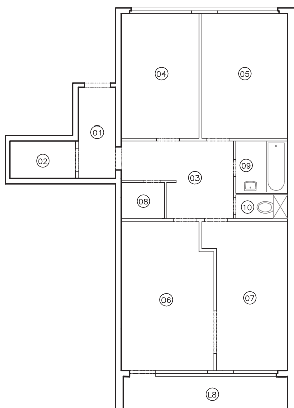
bytová jednotka 687/08
