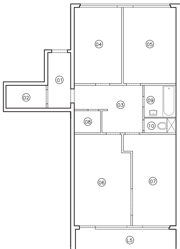
bytová jednotka 689/05
