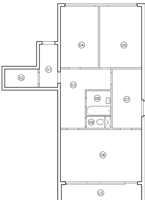
bytová jednotka 686/05
