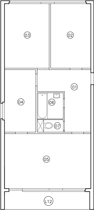
bytová jednotka 689/12
