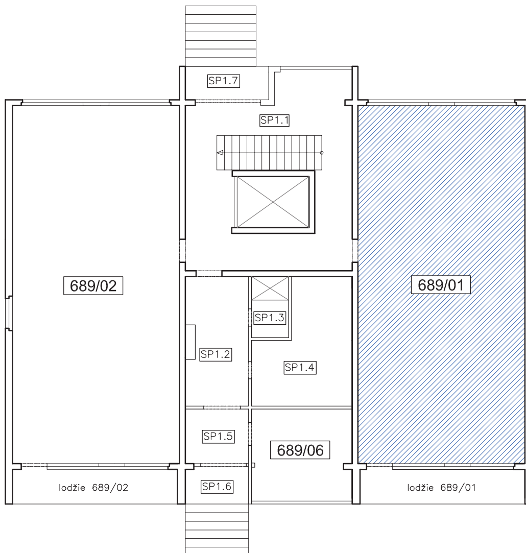
bytová jednotka 689/01
