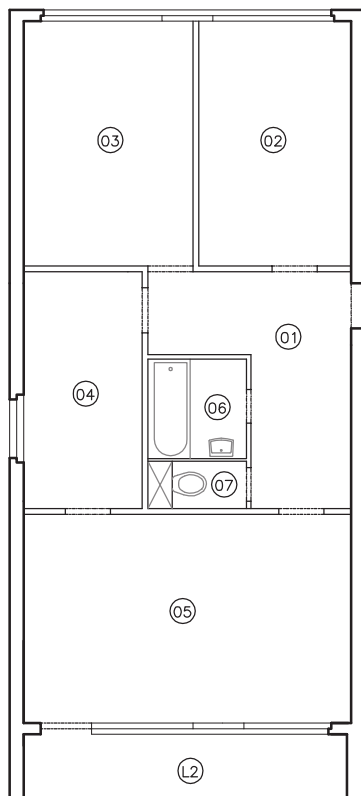
bytová jednotka 689/02
