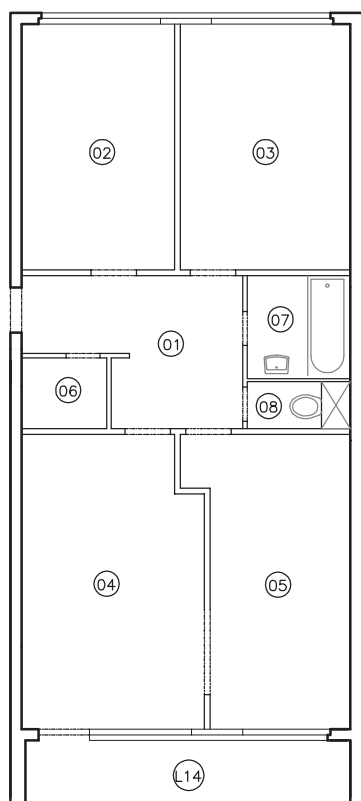
bytová jednotka 687/14
