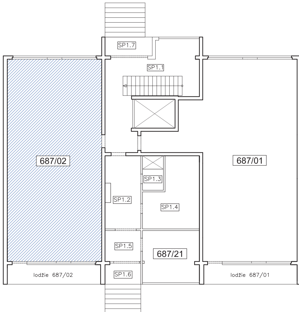
bytová jednotka 687/02
