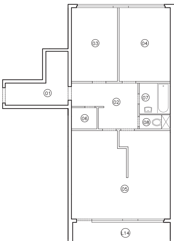
bytová jednotka 688/14
