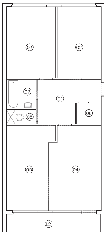
bytová jednotka 687/02
