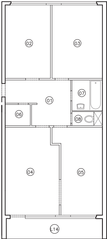
bytová jednotka 689/14
